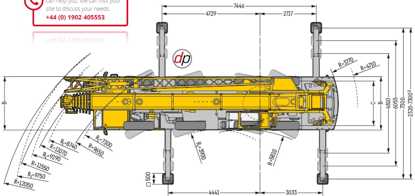
Dimensions
